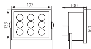
ALIX POWER LED9
