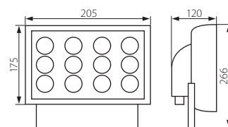
ALIX POWER LED12
