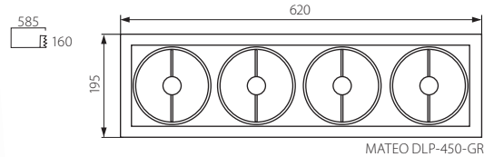
MATEO DLP-450-GR
