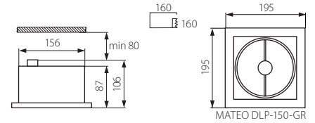
MATEO DLP-150-GR
