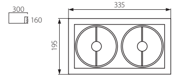
MATEO DLP-250-GR
